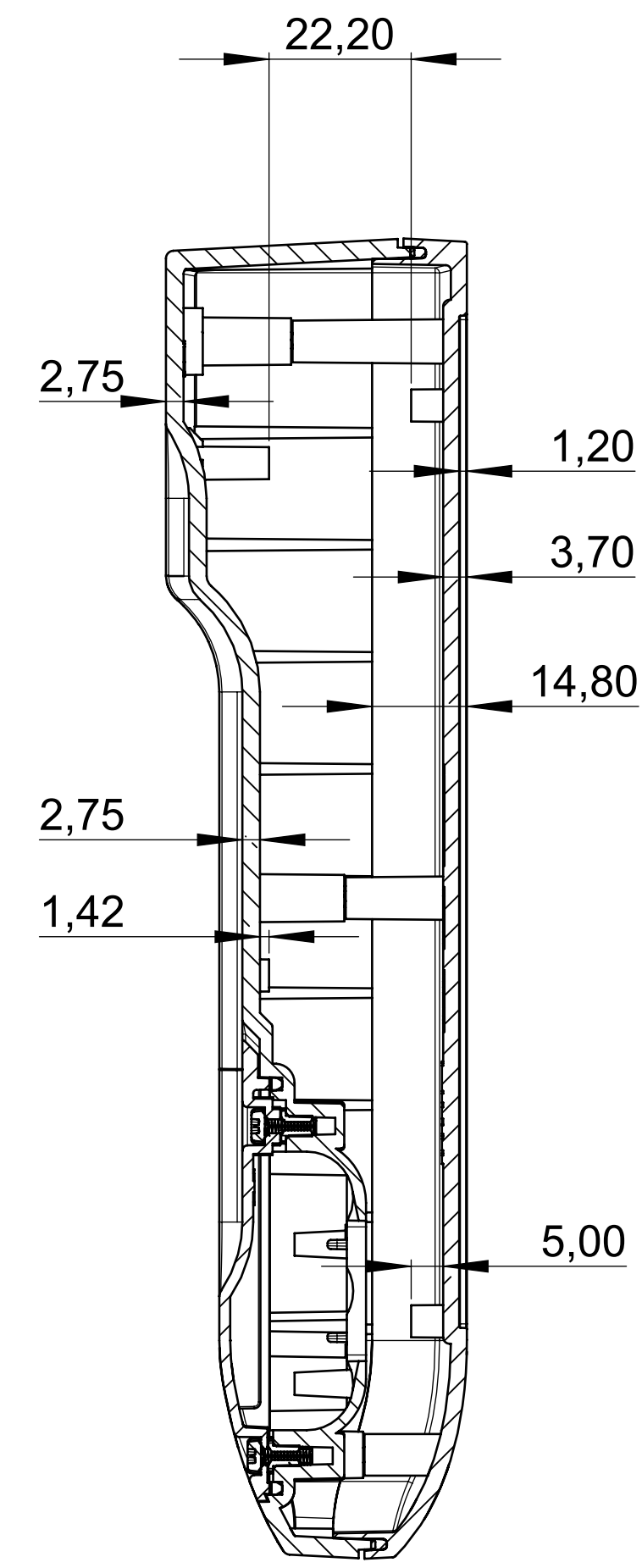
Schnitt A-A Section A-A
