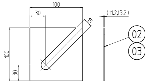
架台用ライナー-外觀寸法 (1 : 4)
