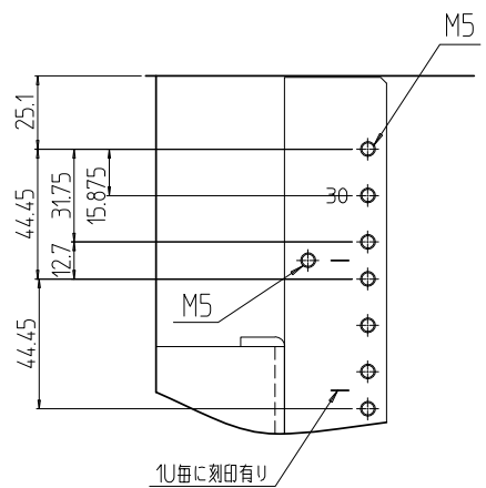
A部詳細 (1 : 3)
