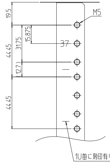
B部詳細 (1 : 2)
