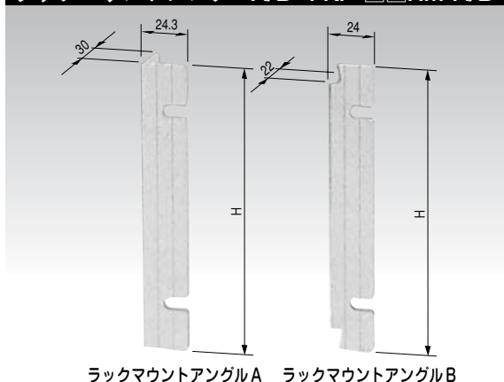
ラックマウントアングルA ラックマウントアングルB
