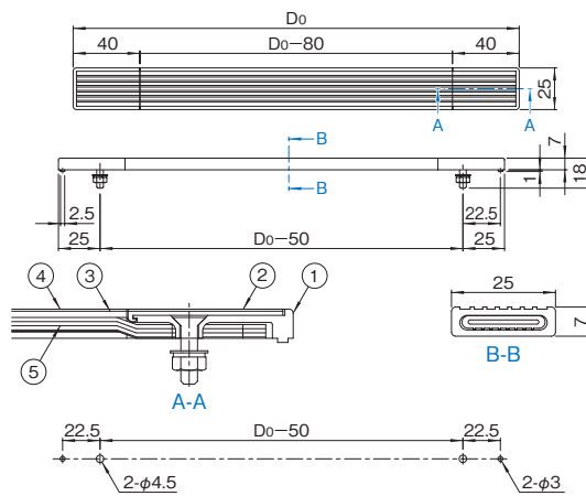
取付穴寸法詳細
