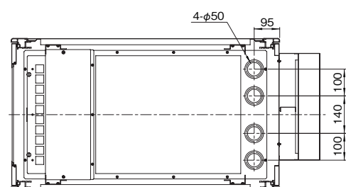
B-B断面
