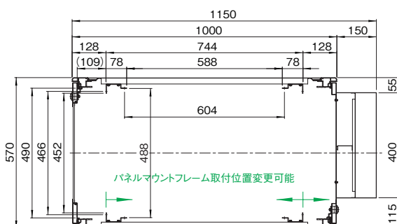
A-A断面
