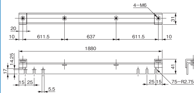
標準取付位置 ラック側面(中間横ハリ)
