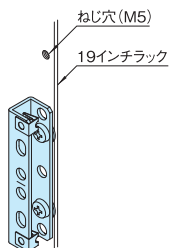
標準取付位置 19インチパネルマウント部
