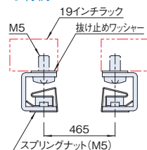
取付例
