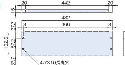
RBP-1348F-N□ (EIA)
