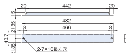
RBP-0448F-N□ (EIA)
