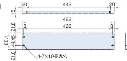
RBP-0848F-N□ (EIA)
