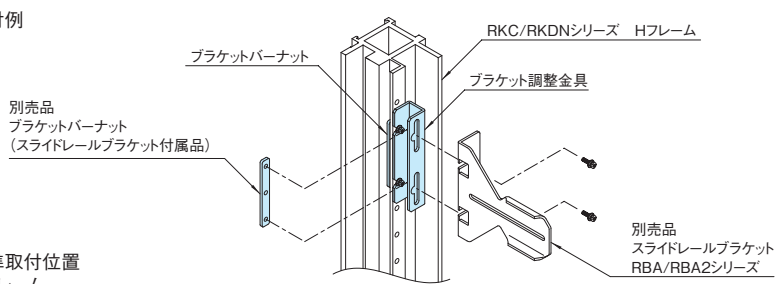
取付例
