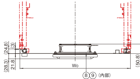
A-A ※防塵ラックDPR2シリーズ W600またはW700 H1514以下の適合機種の場合
