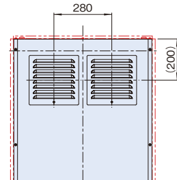
防塵ラックDPR2シリーズ W700 H1764以上の適合機種の場合
