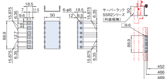
取付例
