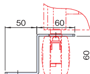
キャスター側面に取り付ける場合
