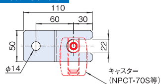
キャスター側面に取り付ける場合
