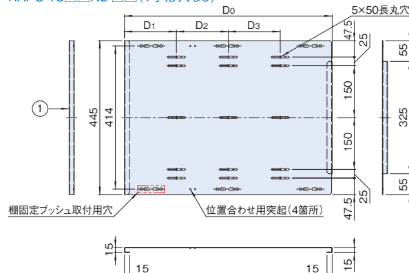
RAPS-15□□NL-□□ (T字形穴なし)
