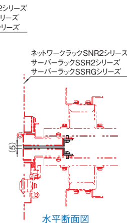
水平断面図
