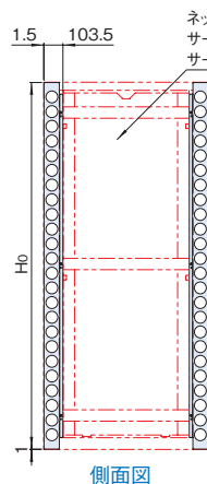
側面図
