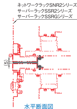
水平断面図
