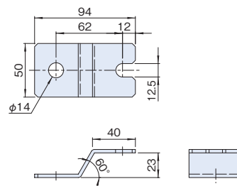
標準取付位置 ラック下面四隅
