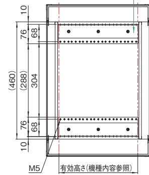
ラック前面側 B-B
