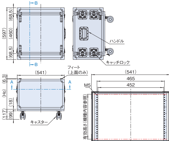
7U以上の機種
