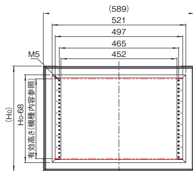
前面(フタを取り外した状態) ※7U以上は後面も同仕様
