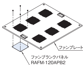
取付例
