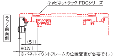
実装例 (水平断面)
