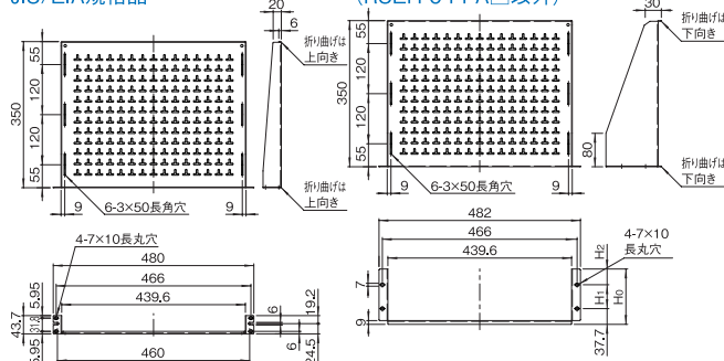
RSEH-044-A□ JIS/EIA規格品
