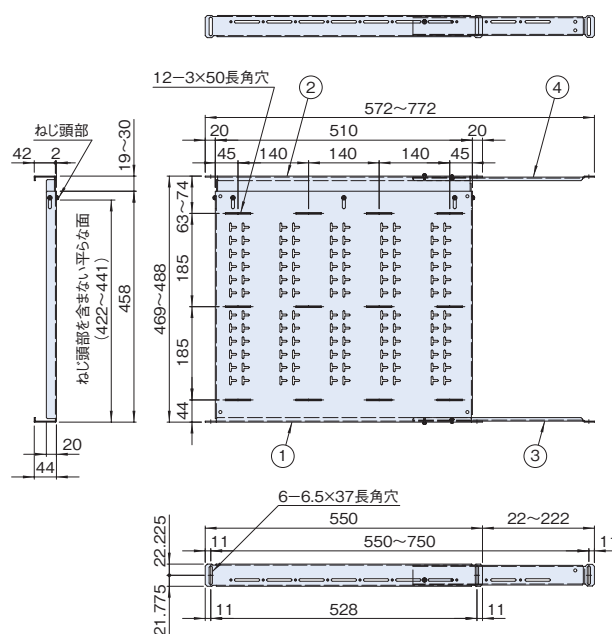
標準取付位置 ラック内部(Hフレーム/マウントフレーム)
