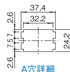
A穴詳細
