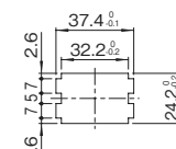
取付穴加工寸法図
