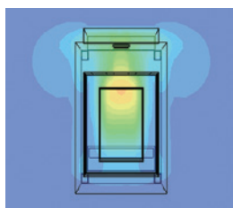
ラックの周りに何も無い状態
