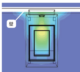
後面を壁につけた状態
