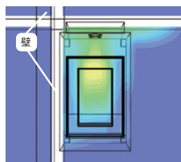
左面と後面を壁につけた状態
