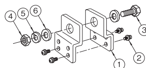
分解図
