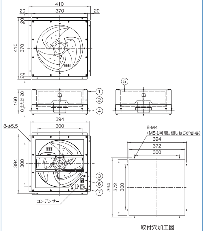
標準取付位置 ラック上面
