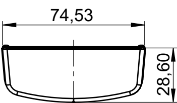
Schnitt C-C
