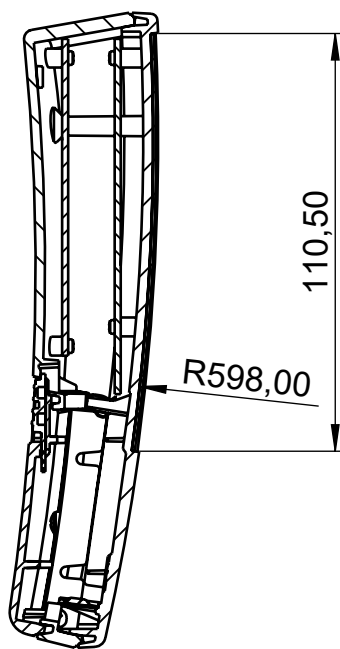
Schnitt C-C
