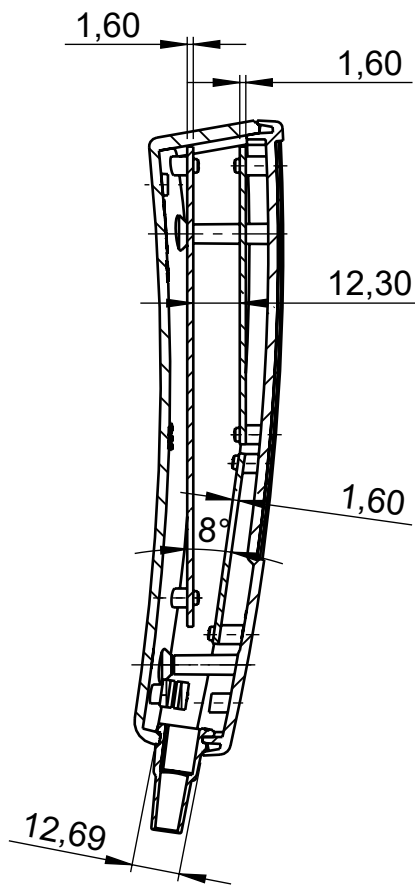
Schnitt B-B
