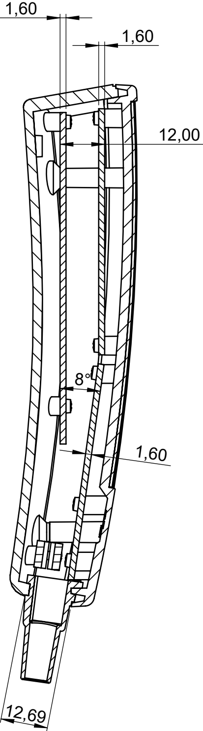
Schnitt B-B
