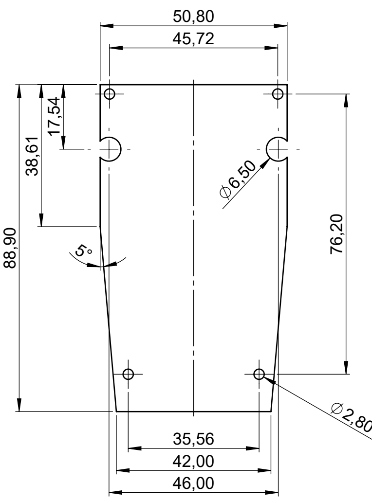
Platine für Unterteil ohne Batteriefach PCB for base part without battery compartment
