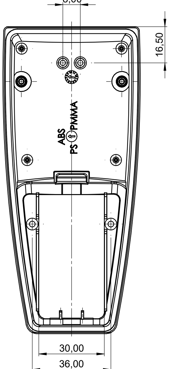
Unterteil mit Batteriefach Base part with battery compartment
