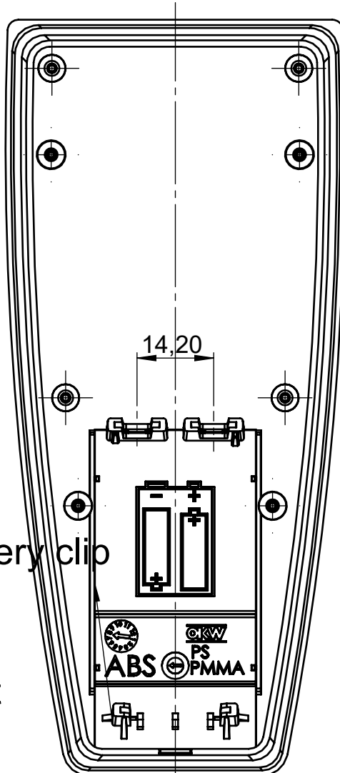
Oberteil Innenansicht Top part inside view
