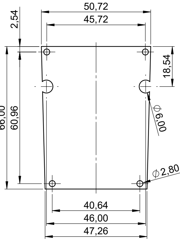
Platine für Oberteil PCB for top part
