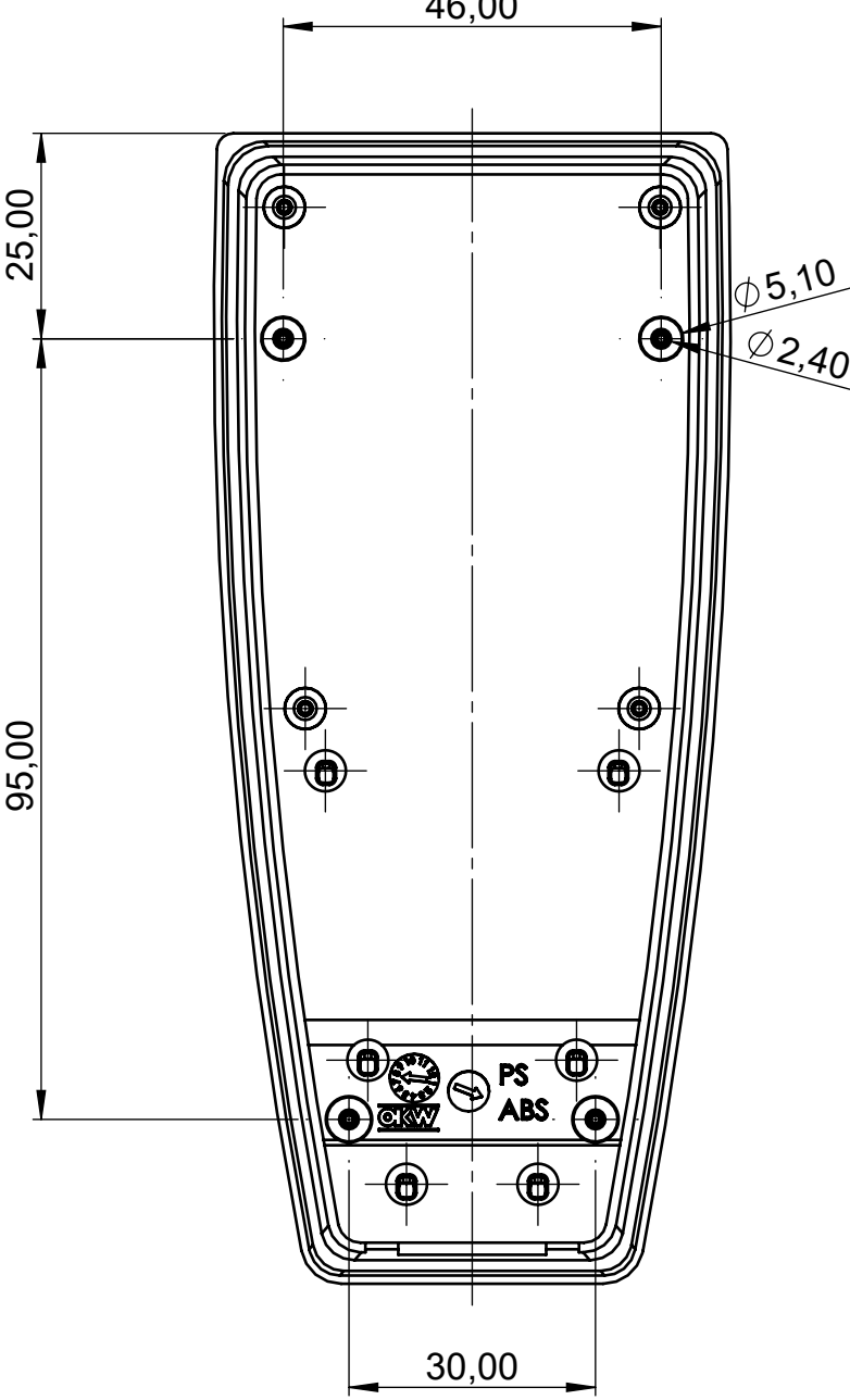
Oberteil Innenansicht Top part inside view
