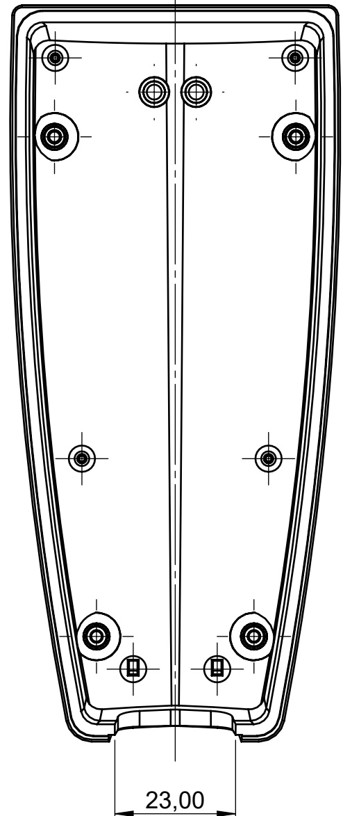
Unterteil mit Aussparung für Kabeltülle Bottom part with cutout for the cable bush
