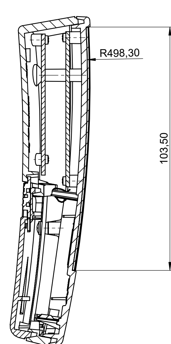
Schnitt C-C
