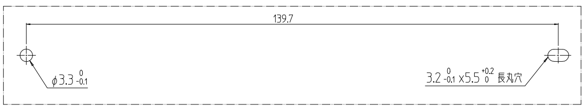
取付穴寸法図
