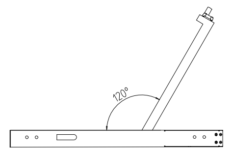
ディスプレイ部を最大限開いた状態 (1:10)
