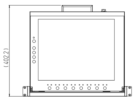
ディスプレイ部を開いた状態(90°) (1:10)
