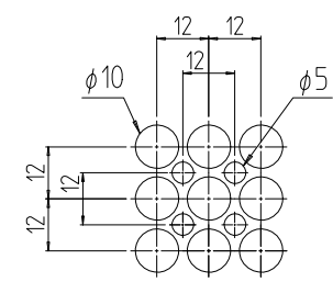
パンチング部詳細 (1 : 2)
