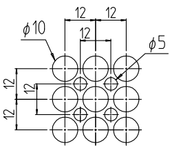
パンチング部詳細 (1 : 2) 開口率 約68%
