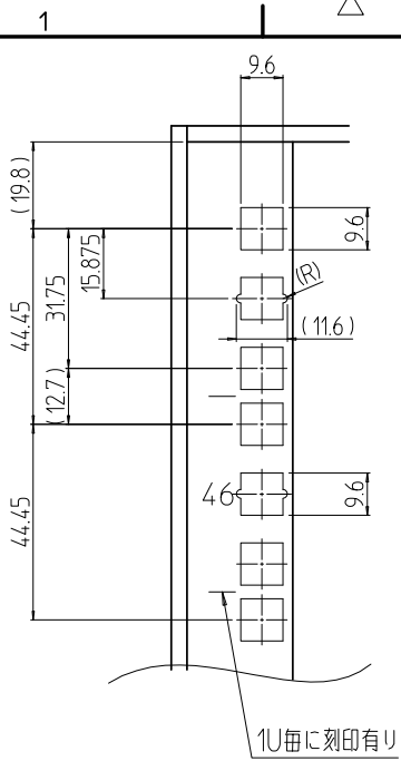
A部詳細 (1 : 2)
