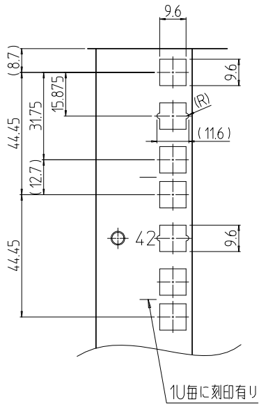
A部詳細 (1 : 2)
