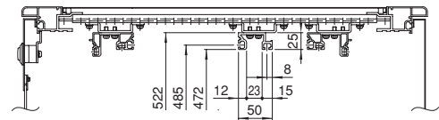
取付例 水平断面図
