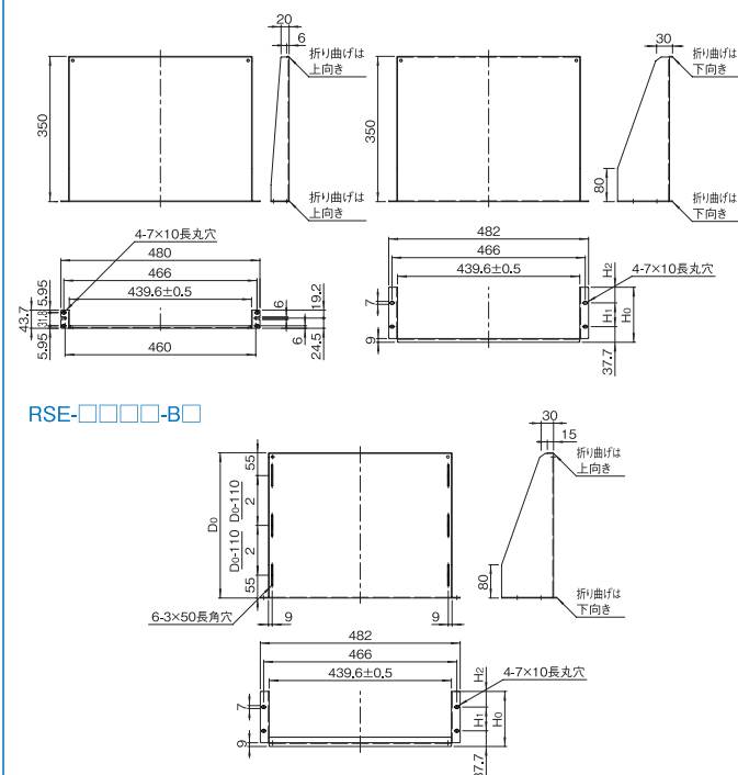
RSE-044-A□ JIS/EIA規格品
