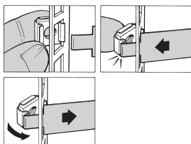
取付例
